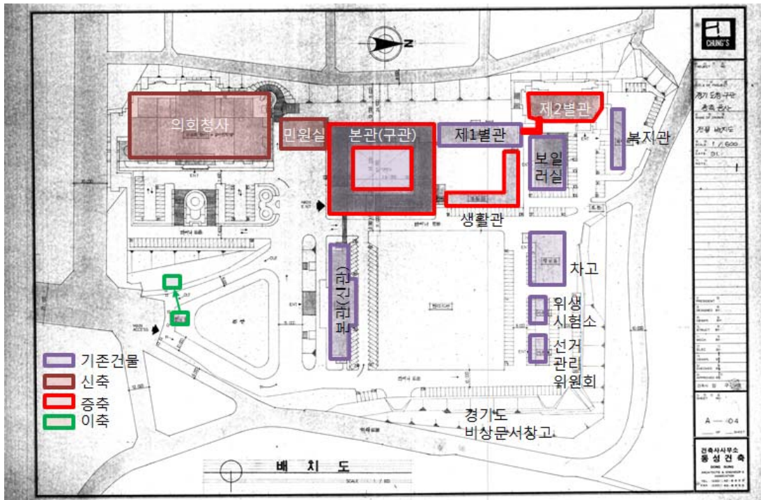
1991년대 초 경기도청 배치 (『경기도청구관 증축공사』 배치도(1991) 위 편집)
