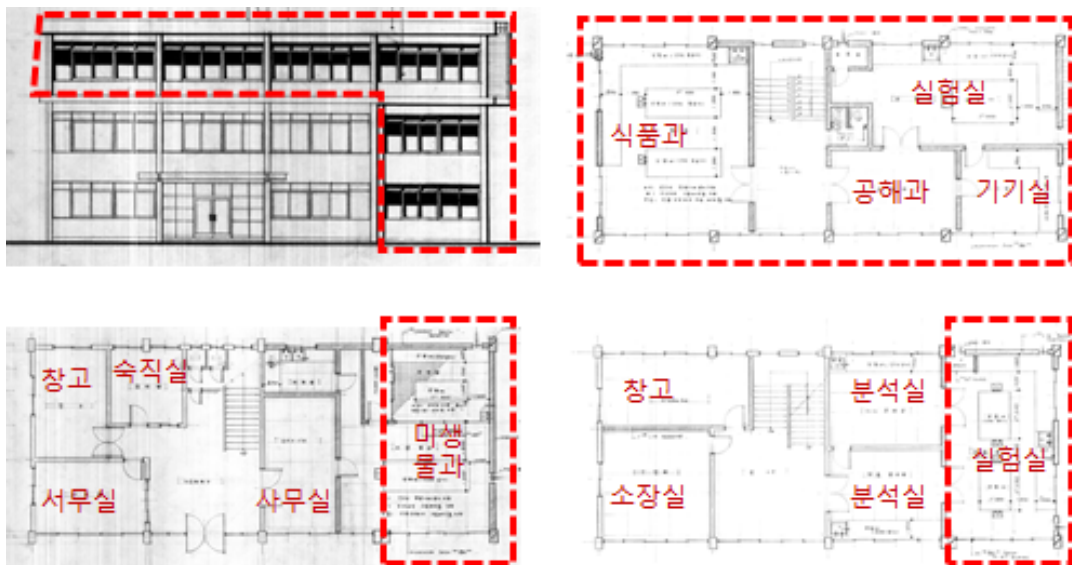
위생시험소 증축공사 도면 (경기도청 소장 <경기도 보건연구소 증축공사>) 좌상: 정면도, 좌하: 1층평면도, 우상: 3층평면도, 우하: 2층평면도
