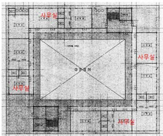
본관(구관) 4층 증축설계 평면도(1991년)
