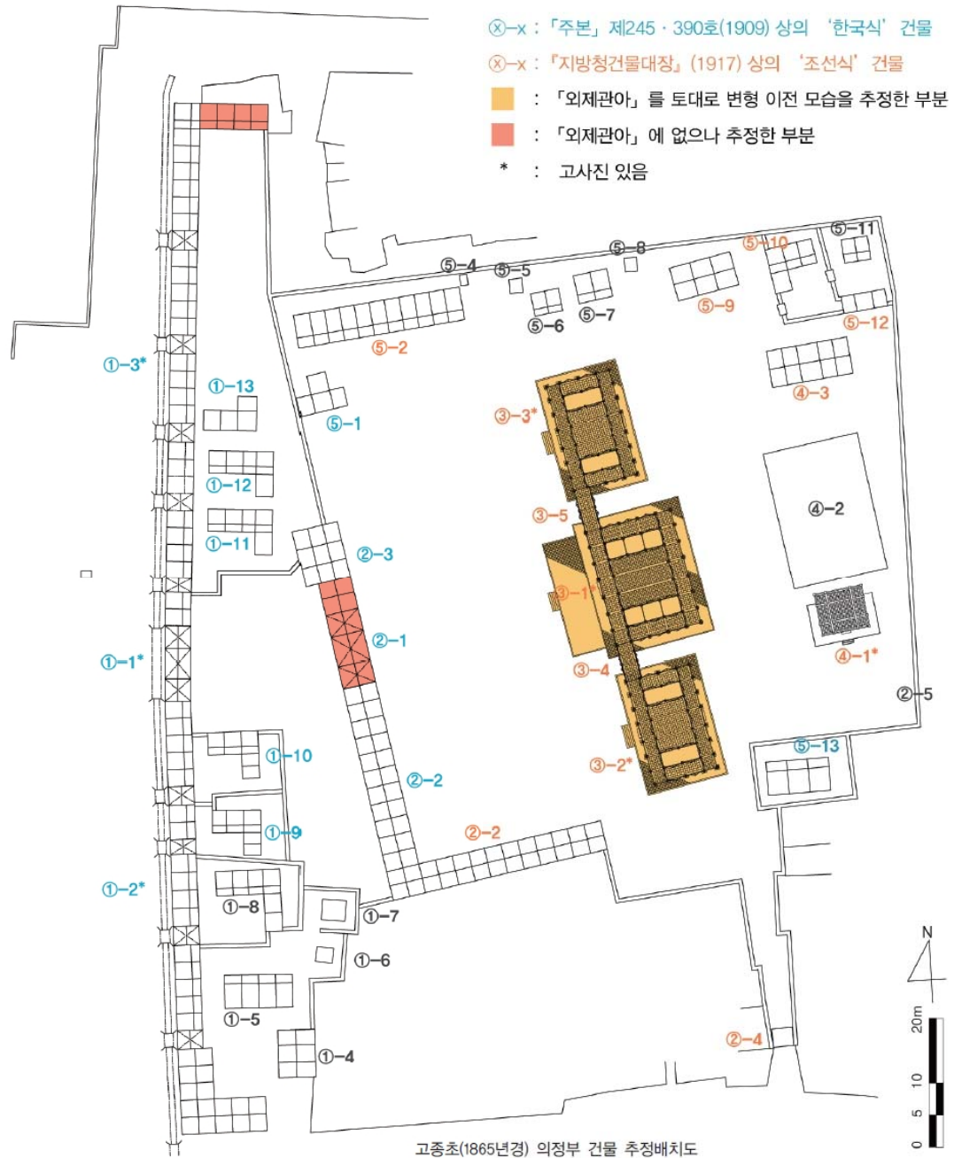
고종초(1865년경) 의정부 건물 추정배치도 (서울특별시·(재)역사건축기술연구소, 『의정부터 정비 및 활용방안 마련 종합학술연구』, 2016.)
