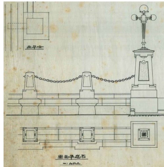
전면 담장 (『내부청사문및석장신설세상도』, 1909~1910 추정, 국가기록원 소장)
