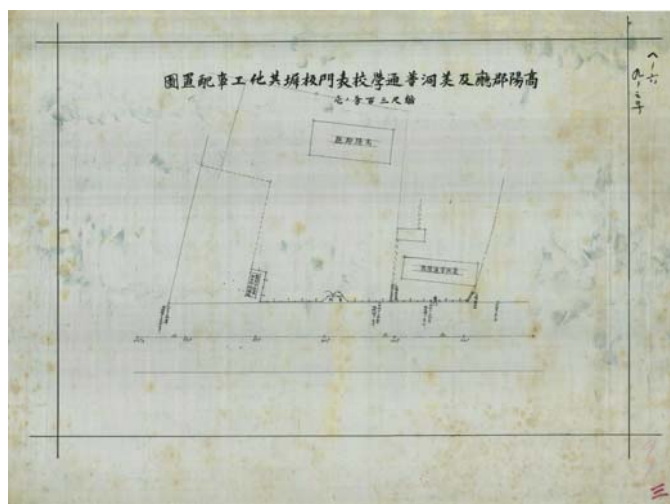
고양군청사급미동보통학교표문판벽기타공사배치도, 국가기록원 소장, 표문설계도, (추정)1910년대, 국가기록원 일제시기 건축도면 콘텐츠
