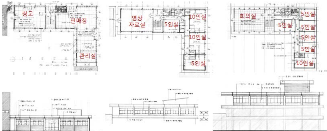
생활관 신축 및 증축공사 도면
