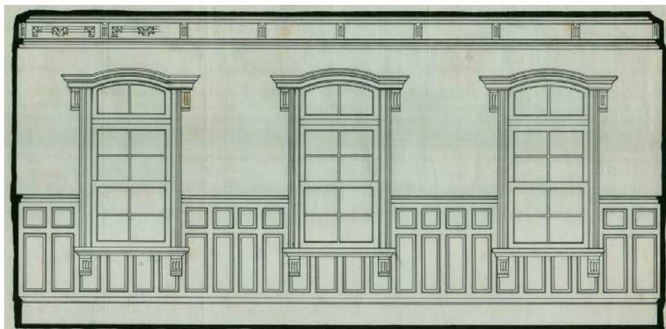
대신실 정면 입면 (「내부청사신축공사설계도」, 1909~1910 추정, 국가기록원 소장)
