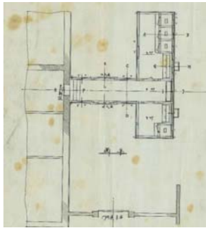
변소의 평면(「경기도청부속측급도랑하신축지도」, 1911년경 추정, 국가기록원 소장)
