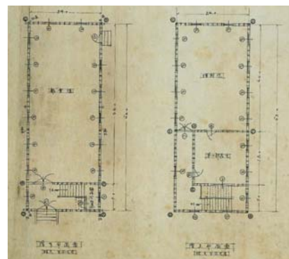
신축된 권업계·이재계 건물 평면 (「경기도청사증축공사설계도」, 1916년경, 국가기록원 소장)
