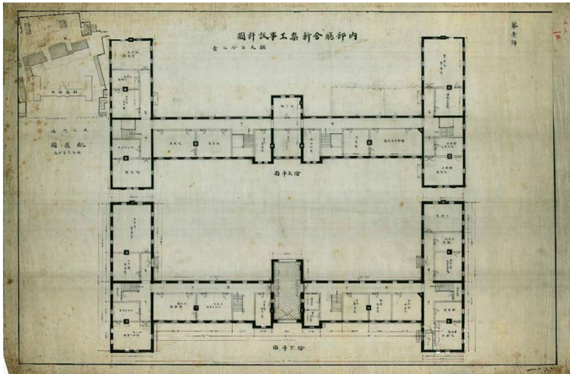
내부 청사 층별평면도 (「내부청사신축공사설계도 1」, 1909~1910 추정, 국가기록원 소장)
