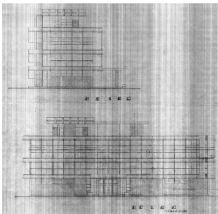
적십자 경기도지사 입면도 (경기도청 소장 <적십자 경기도지사 신축공사>)
