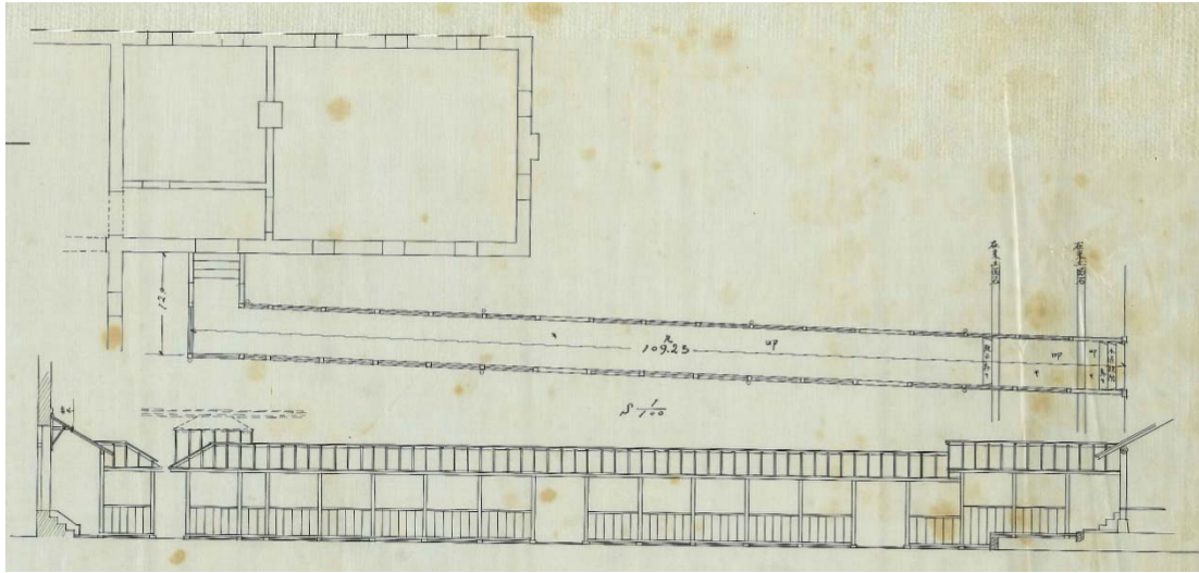
복도각의 평면 및 입면 (「경기도청부속측급도랑하신축지도」, 1911년경 추정, 국가기록원 소장)
