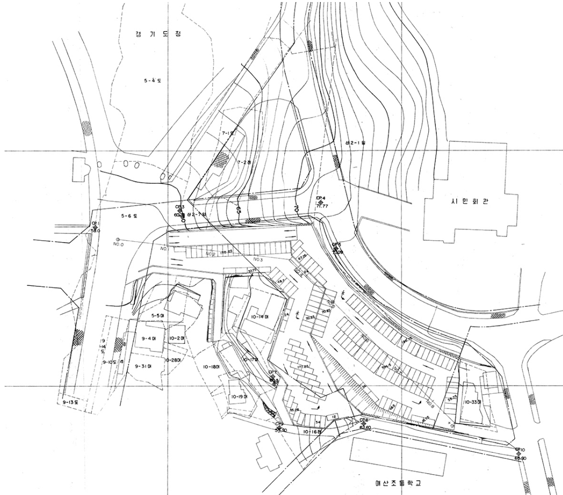
경기도청 옥외주차장 설치공사 배치도
