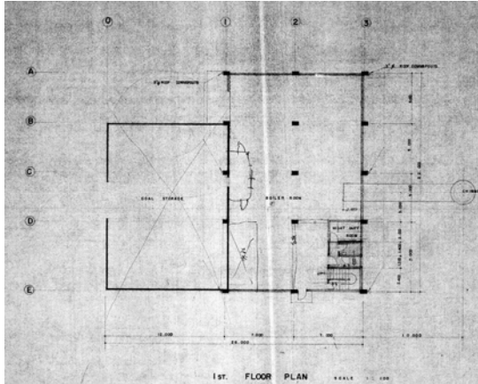
최초 보일러실 평면도 (우:보일러실, 좌:석탄창고) (경기도청 소장 <기관실 건축도>)
