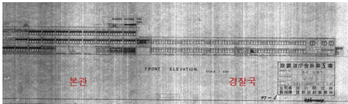
경기도청 본관(구관)과 경찰국 1층 정면도 (경기도청 소장 <본관·경찰국 입면도>)
