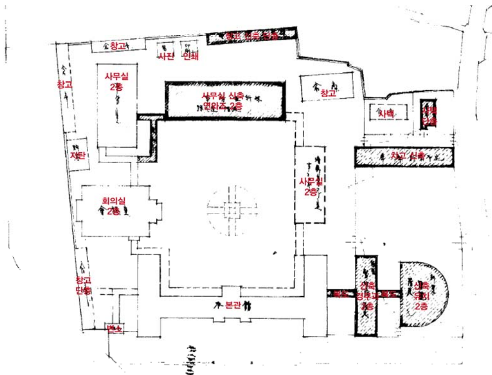
1930년에 작성된 증개축 계획안 (경기도, 「소화육년도세출계획서」, 국가기록원, CJD0002793)
