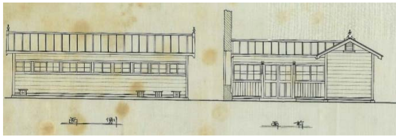
변소의 입면 (「경기도청부속측급도랑하신축지도」, 1911년경 추정, 국가기록원 소장)
