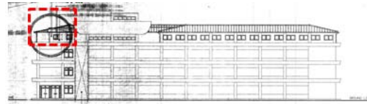
본관(구관) 4층 화장실 증축설계 동측면도(1992년)
