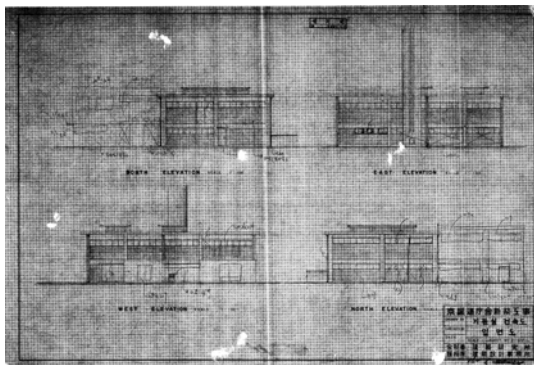
최초 보일러실 입면도 (증축계획이 스케치로 표현) (경기도청 소장 <기관실 건축도>)
