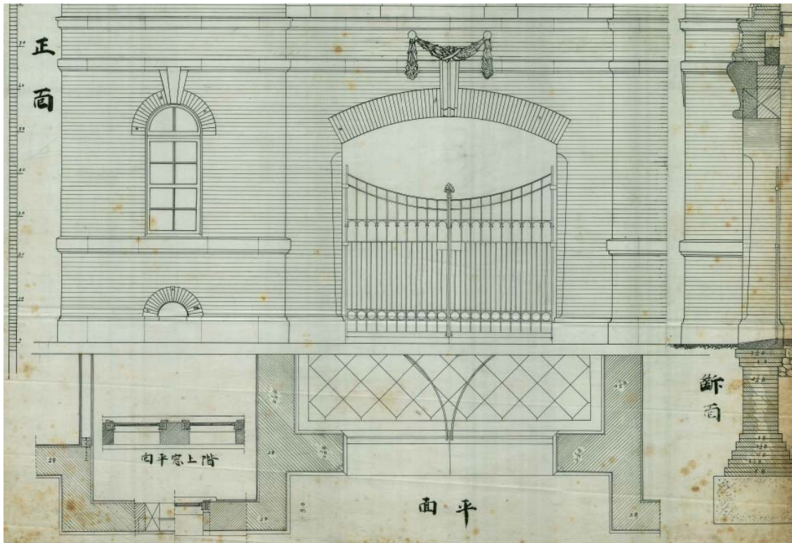
청사의 정면 주출입구의 입면도 및 평면도 (「내부청사신축공사설계도」, 1909~1910 추정, 국가기록원 소장)
