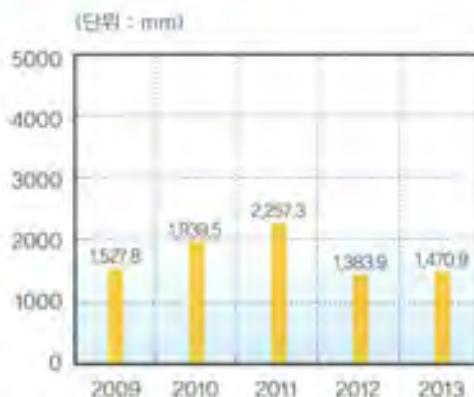
연별 강수량
