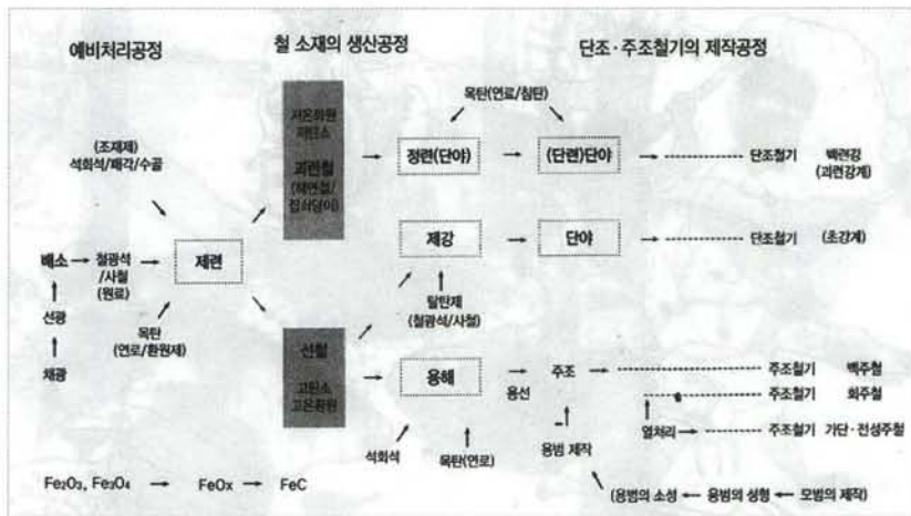
[그림 1] 製鐵과 製鋼의 프로세스(『한반도의 제철유적』, 한국문화재조사연구기관협회, 2012, 11)
