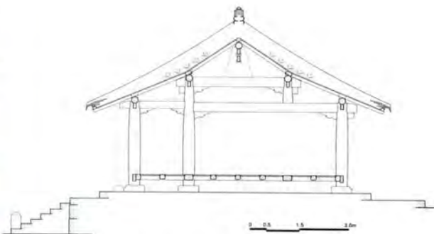
그림 49. 강당 종단면도 (『북한문화재해설집 III』, 264쪽)
