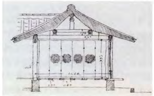
그림 52. 자남동 조씨택 사랑채 단면도 (1933년 작도, 1:30으로 추정)
