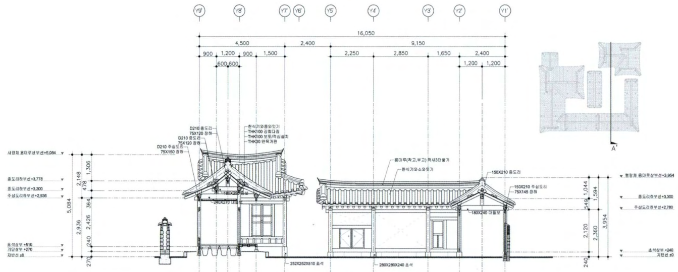
남-북 단면도 2
