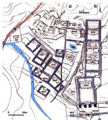
그림 5. 궁궐 배치도 세부 (홍영의, 앞의 글, 46쪽, 재인용)
