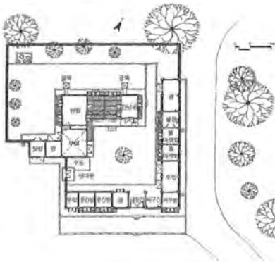
그림 32. 경기도 민가 (양주 백수현가옥)
