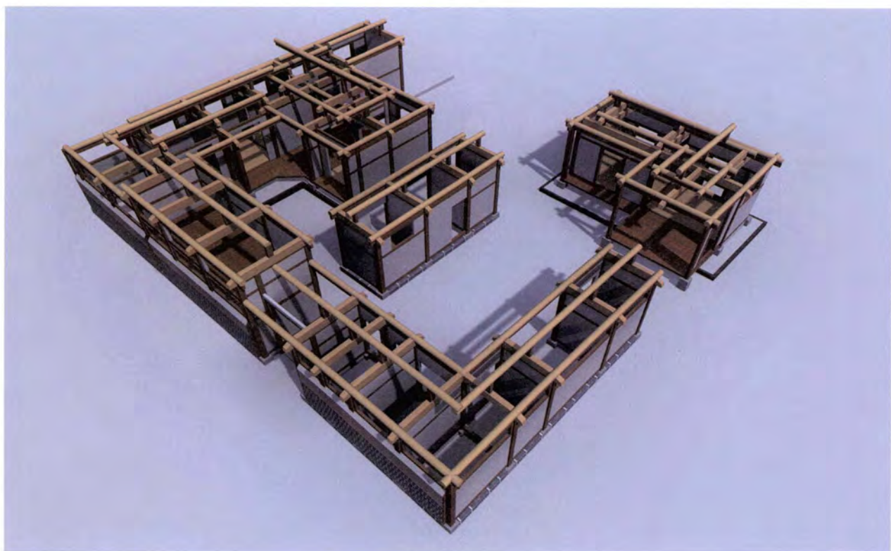
화방벽 설치
