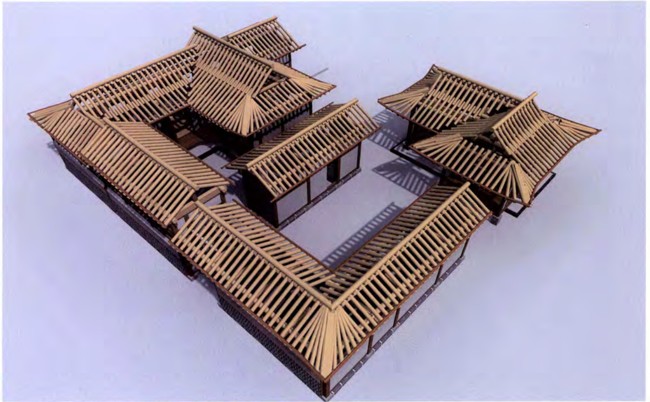
서까래 조립
