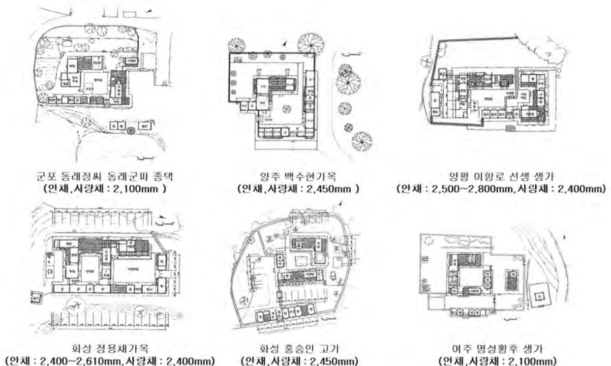
그림 35. 경기도 민가의 평면도와 주칸
