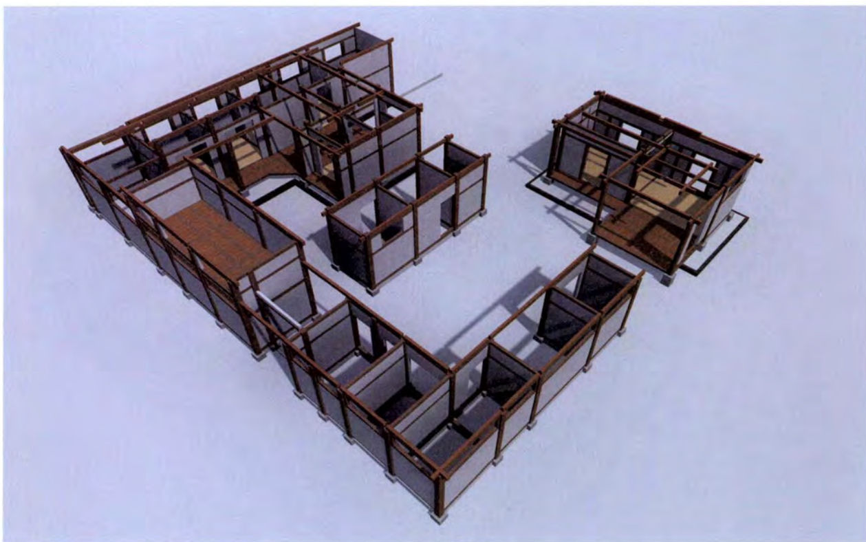
장여 조립
