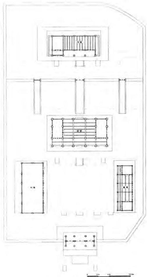
그림 45. 송양서원 배치도 (『북한문화재해설집 III』, 261쪽)
