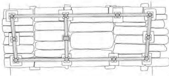
그림 52. 선죽교 평면도 및 단면도 (『북한문화재해설집 1-석조물편』, 353쪽)
