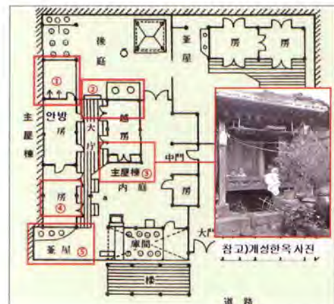
1997년 평면
