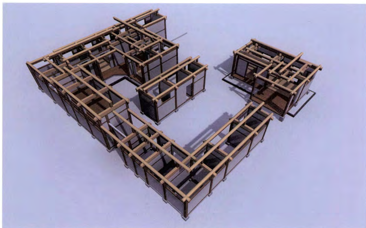
보 조립
