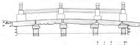
그림 52. 선죽교 평면도 및 단면도 (『북한문화재해설집 1-석조물편』, 353쪽)
