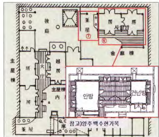
1997년 평면
