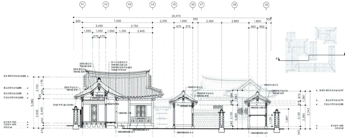
동-서 단면도 1
