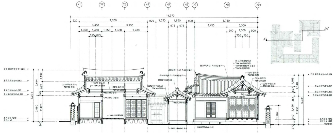
동-서 단면도 2
