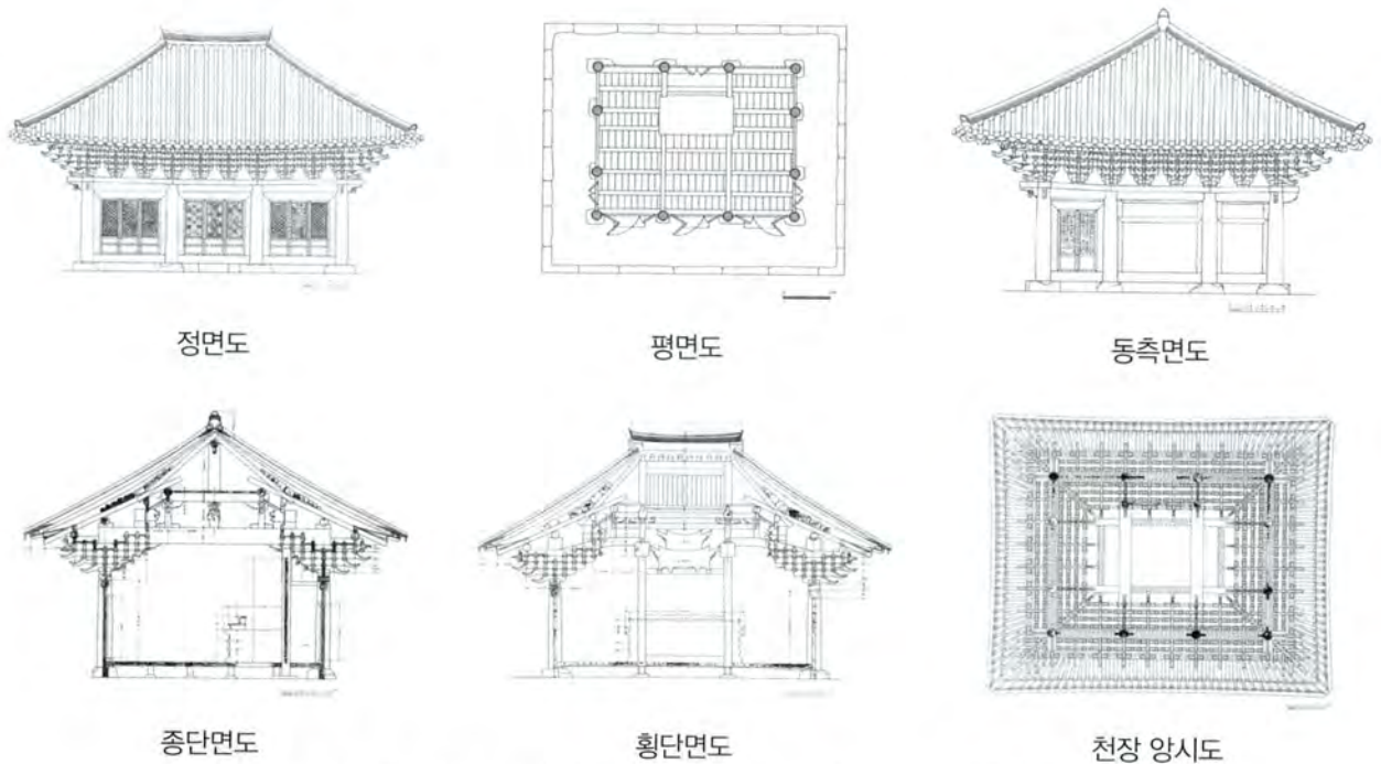
그림 14. 관음사 대웅전 실측도면(『북한문화재해설집 II』, 32~33쪽)
