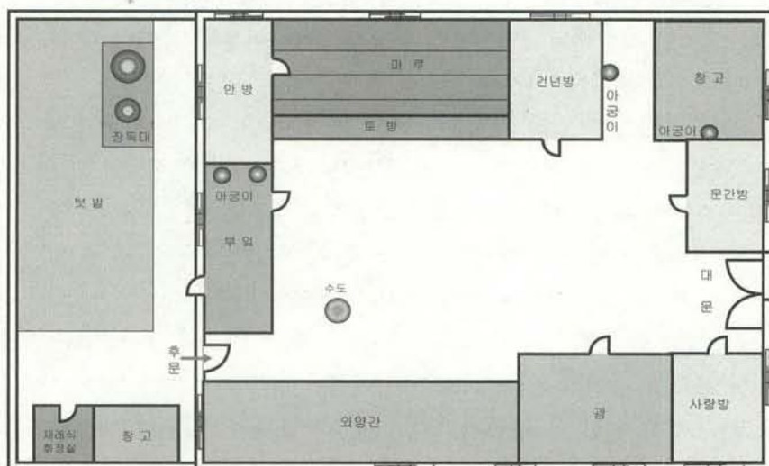
조학년씨덕 집 평면도 - 과거
